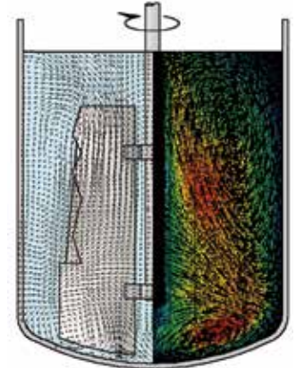
P.T.V. 流動解析結果と C.F.D. による数値シミュレーション結果の比較
