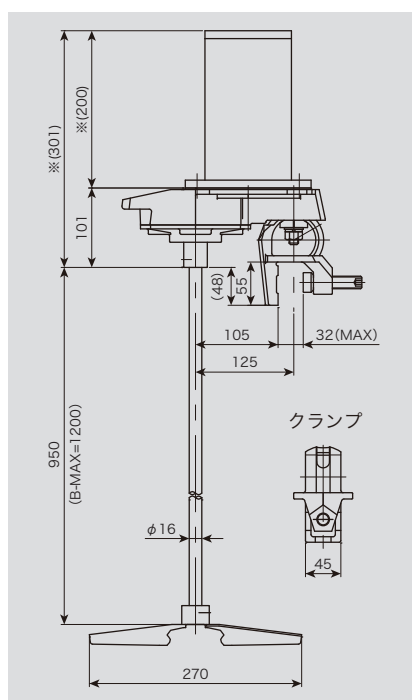
寸法図
