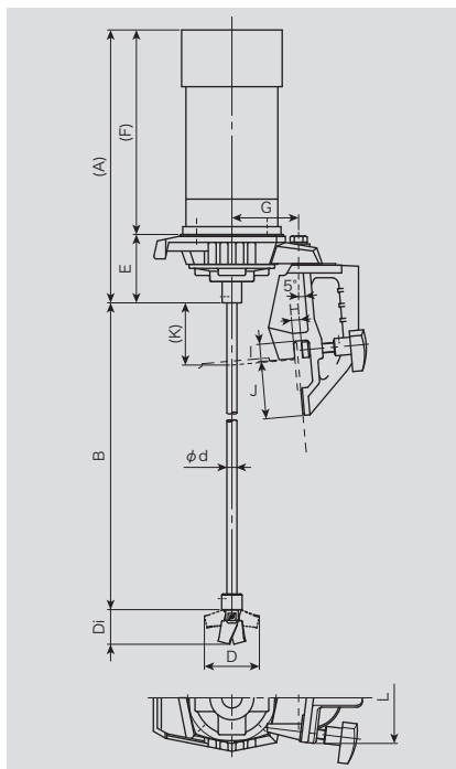
寸法図
