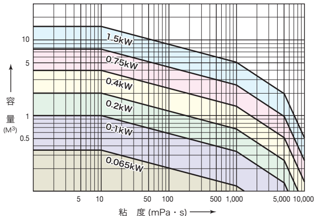
■ 液粘度で検討 (A720 の場合)
