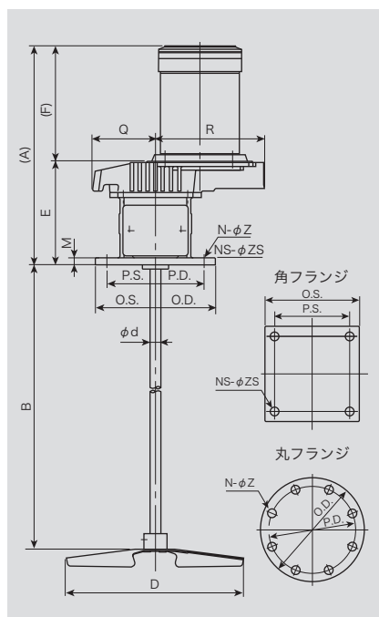
寸法図
