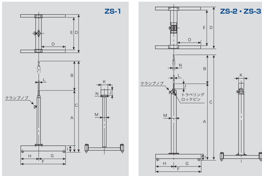
寸法表（手動昇降式）
