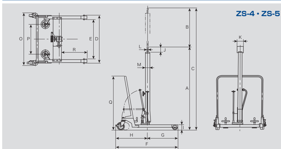
寸法表（油圧昇降式）
